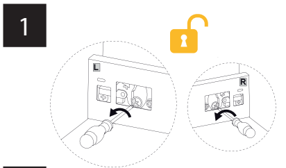
Regolazione dei cassetti / Drawer adjustment Schubladenverstellung
