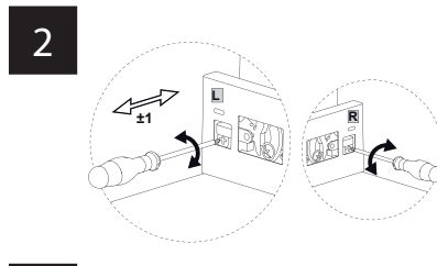
Regolazione dei cassetti / Drawer adjustment Schubladenverstellung
